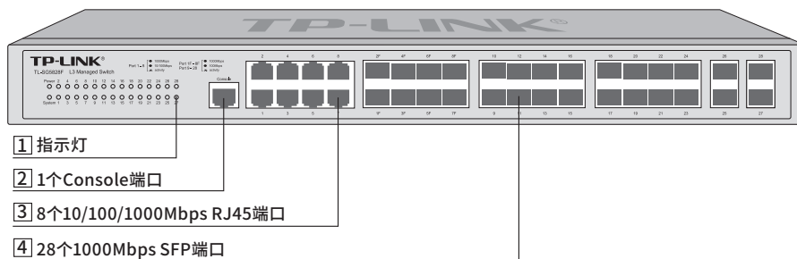
图1-3 TL-SG5828F前面板示意图
