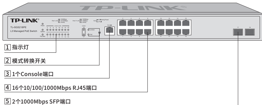
图1-11 TL-SG5218PE前面板示意图
