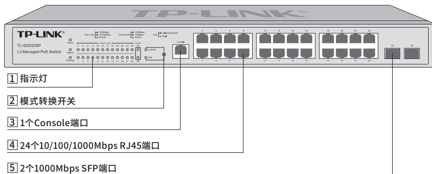
图1-10 TL-SG5226P前面板示意图
