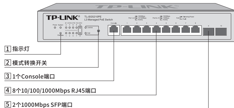
图1-12 TL-SG5210PE前面板示意图
