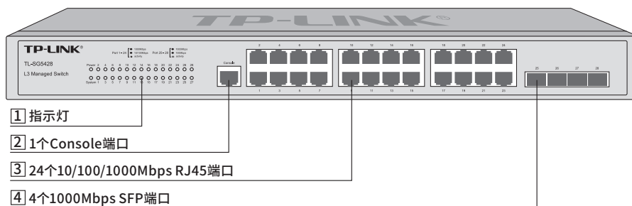
图1-2 TL-SG5428前面板示意图
