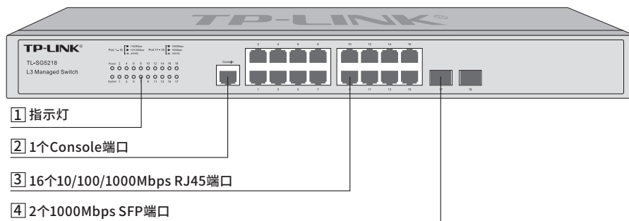
图1-5 TL-SG5218前面板示意图
