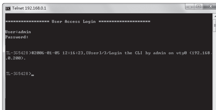
图4-6 登录交换机
