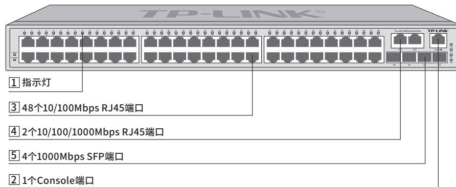
图1-13 TL-SL5452-Combo前面板示意图
