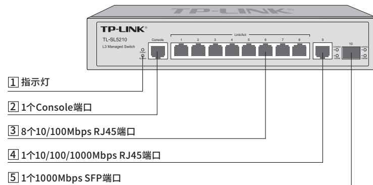
图1-16 TL-SL5210前面板示意图
