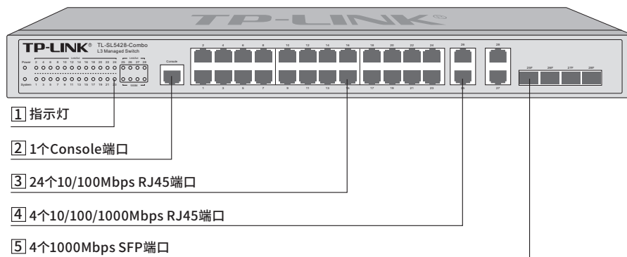
图1-14 TL-SL5428-Combo前面板示意图
