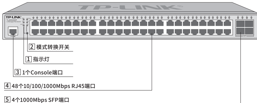
图1-7 TL-SG5452P前面板示意图
