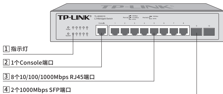
图1-6 TL-SG5210前面板示意图
