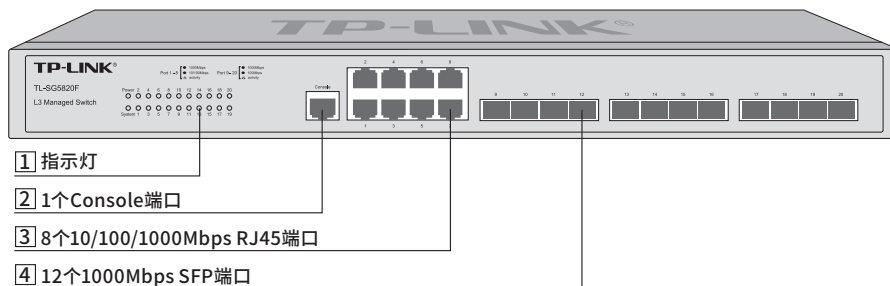
图1-4 TL-SG5820F前面板示意图
