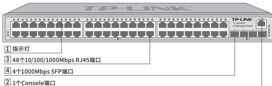
图1-1 TL-SG5452前面板示意图
