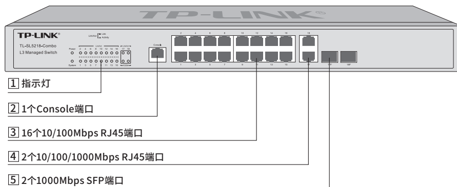
图1-15 TL-SL5218-Combo前面板示意图
