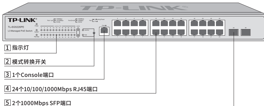
图1-9 TL-SG5226PE前面板示意图
