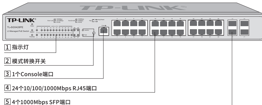
图1-8 TL-SG5226PE前面板示意图
